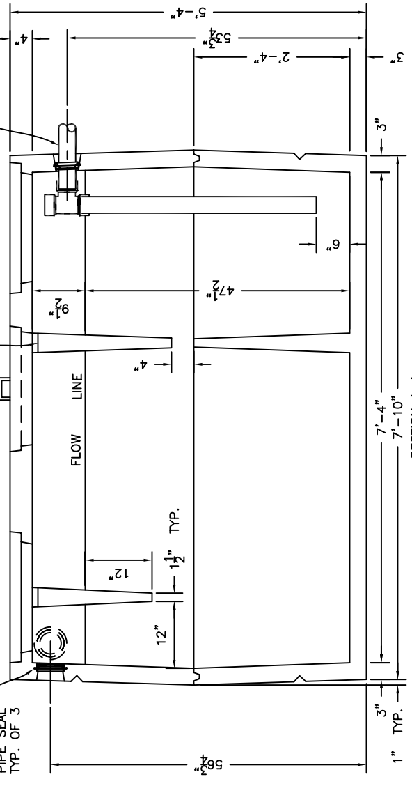
SECTION A-A
