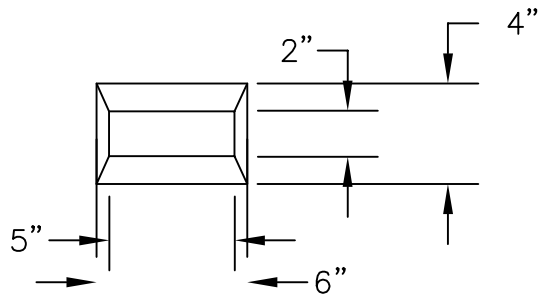
TYP. HOLE DET.
